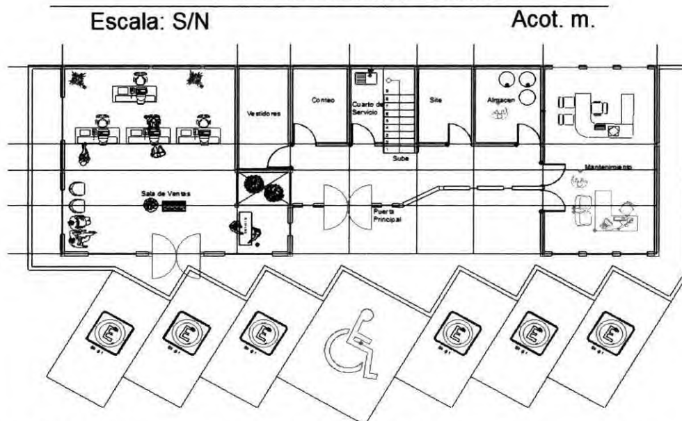
Figura 11. Área de Oficinas de la Estación NATGAS SUR Aguascalientes (Planta Baja y Planta Alta).
