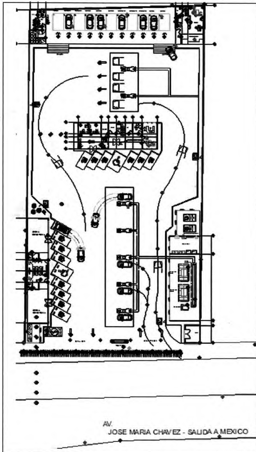
Figura 10. Planta de Conjunto (Proyecto Arquitectónico) de la Estación de NATGAS SUR.
