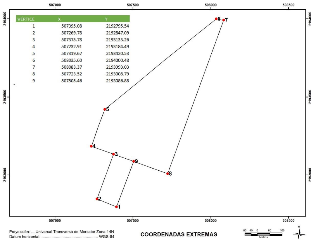
Figura 2.3. Plano de coordenadas de la TPVM.
