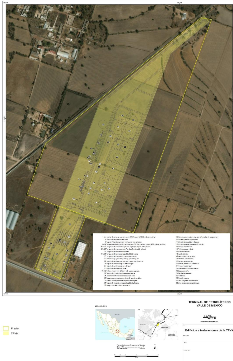
Figura 2.2. Plano de infraestructura de la TPVM.
