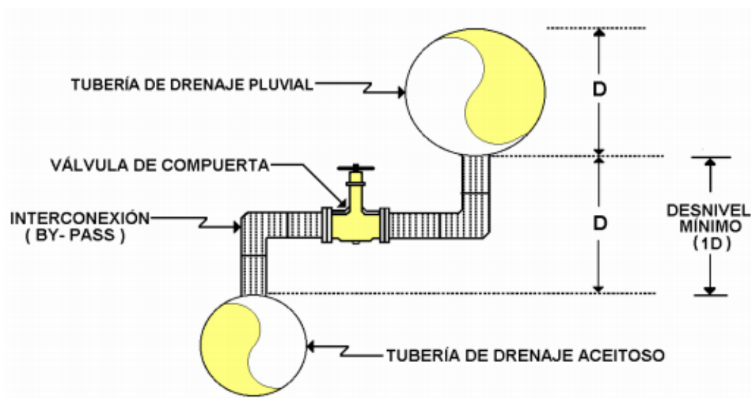
Figura 6.6. Ejemplo de interconexión de drenaje pluvial a aceitoso. Fuente: Pemex, 2008. NRF-015-PEMEX-2008 Modificación 1
