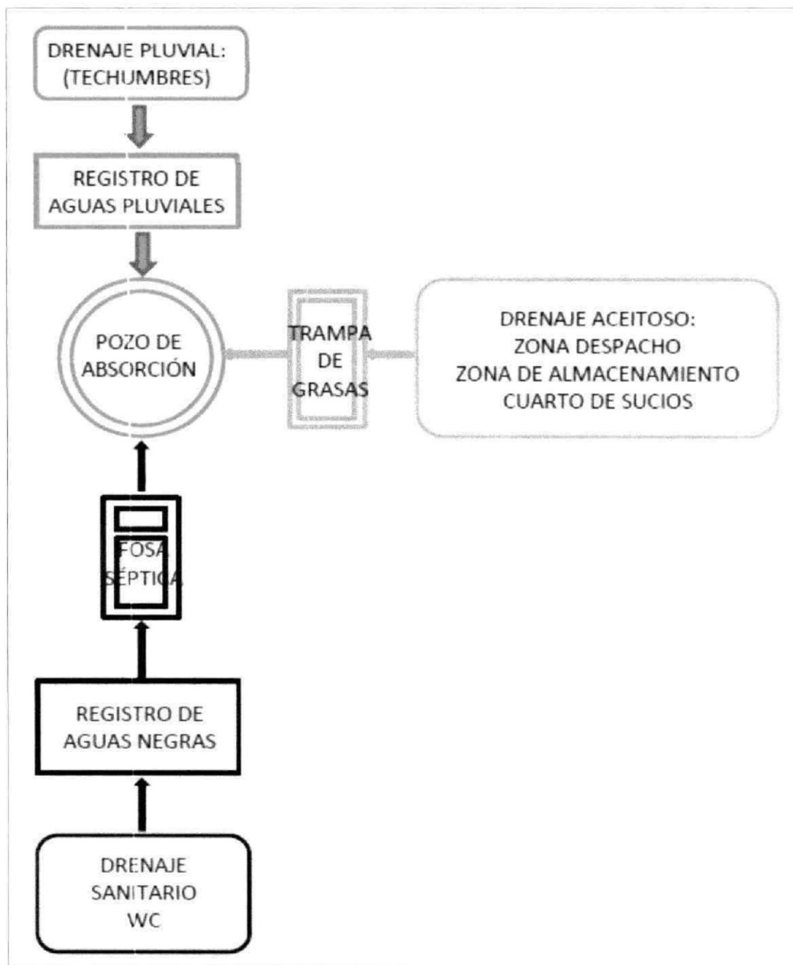
Figura 6. Diagrama de flujo y generación de aguas residuales.
