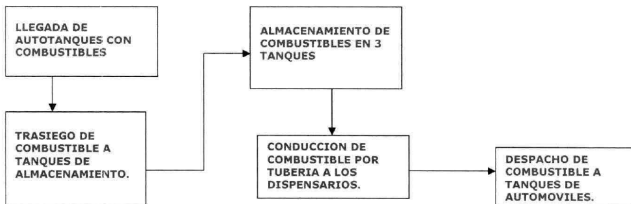
Figura 5. Diagrama de proceso.
