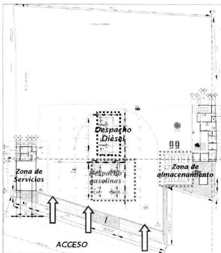
Figura 4. Planta de conjunto.
