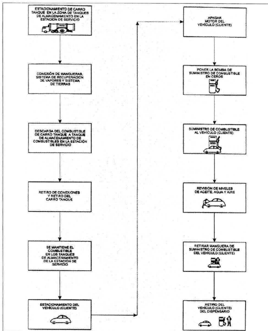
Figura. 3. Diagrama de bloques del proceso operativo de la estación de servicio tipo urbana.
