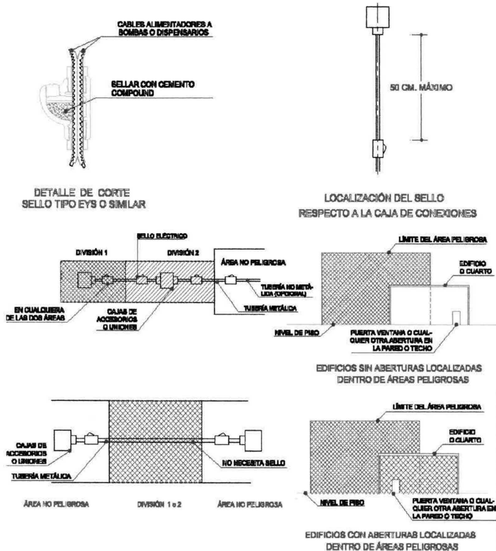
Figura II.8.- Extensión de áreas peligrosas y sellos eléctricos.
