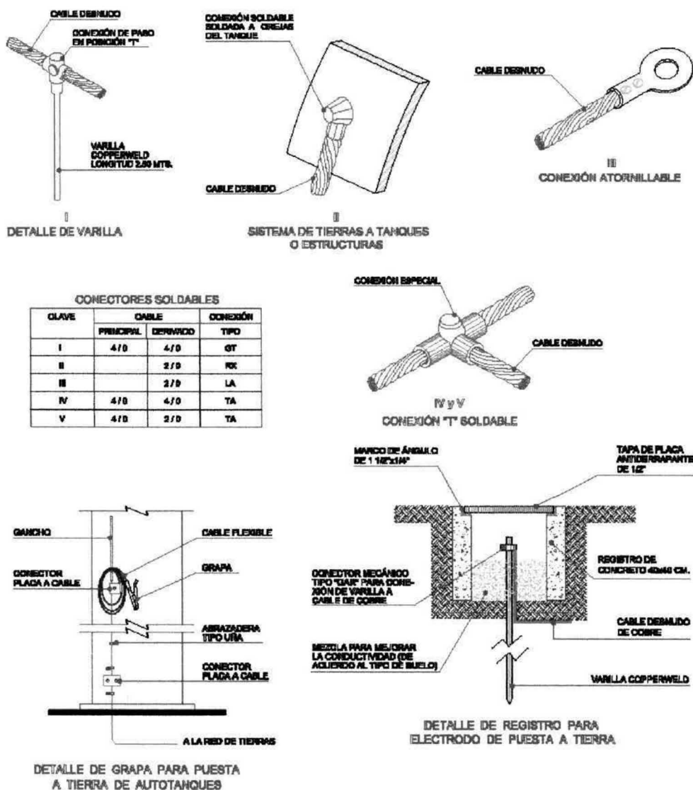
Figura II.9.- Sistemas de tierras.
