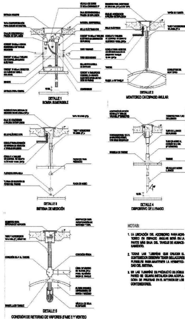
Figura II.10.- Detalles de accesorios para tanques de almacenamiento.
