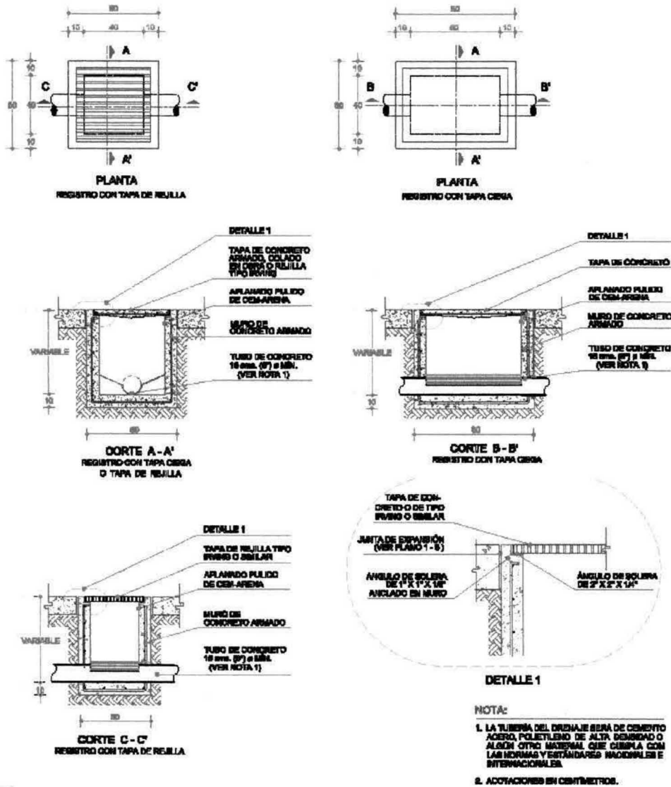
Figura II.5.- Detalle típico para instalación de drenaje.
