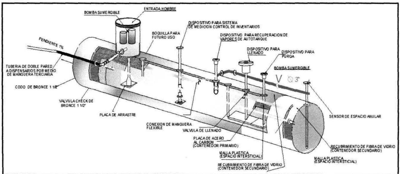
Figura II.1.- Corte esquemático de tanque de doble pared ecológico.
