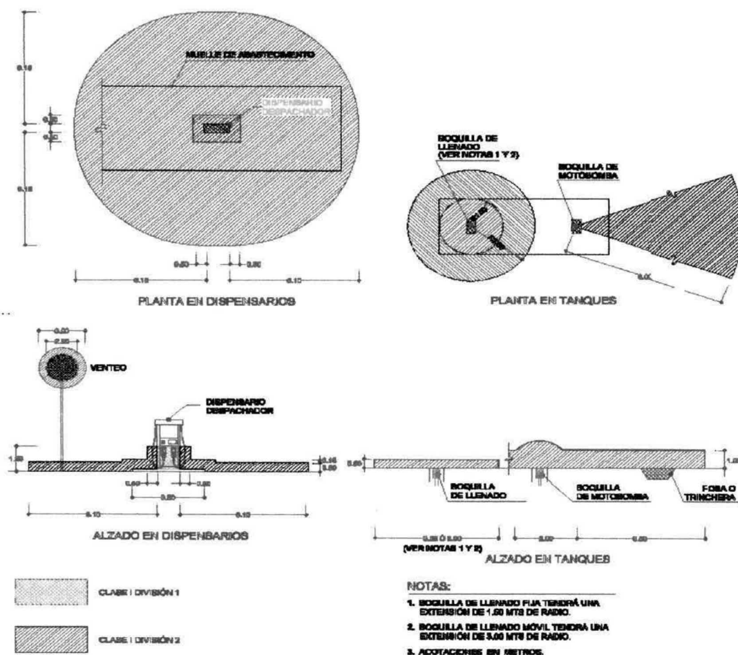
Figura II.7.- Clasificación de áreas peligrosas.
