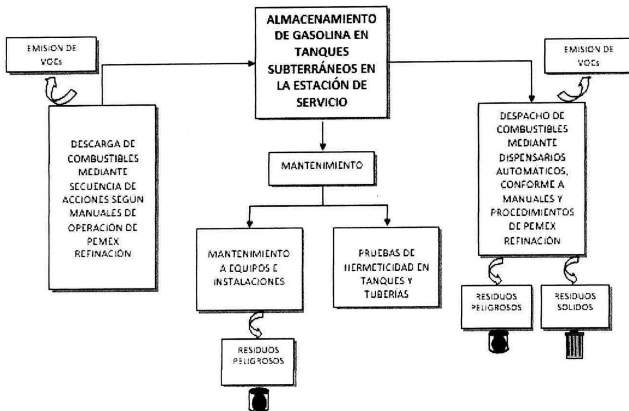
Figura 6. Diagrama de las afectaciones aire, agua y suelo.
