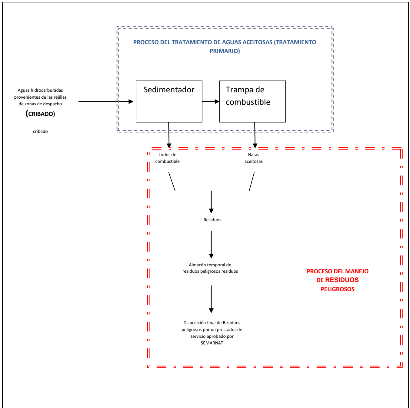
Imagen 5. Diagrama del proceso de aguas hidrocarburadas (aceitosas)
