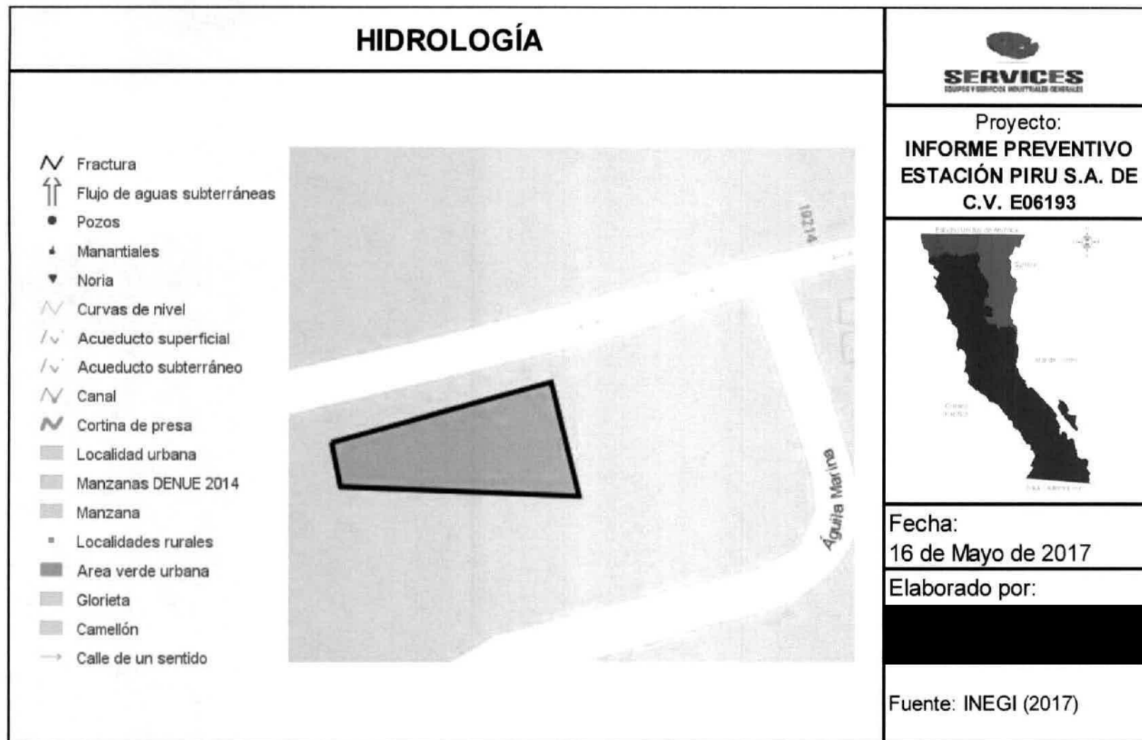
FIGURA 17. HIDROLOGÍA
