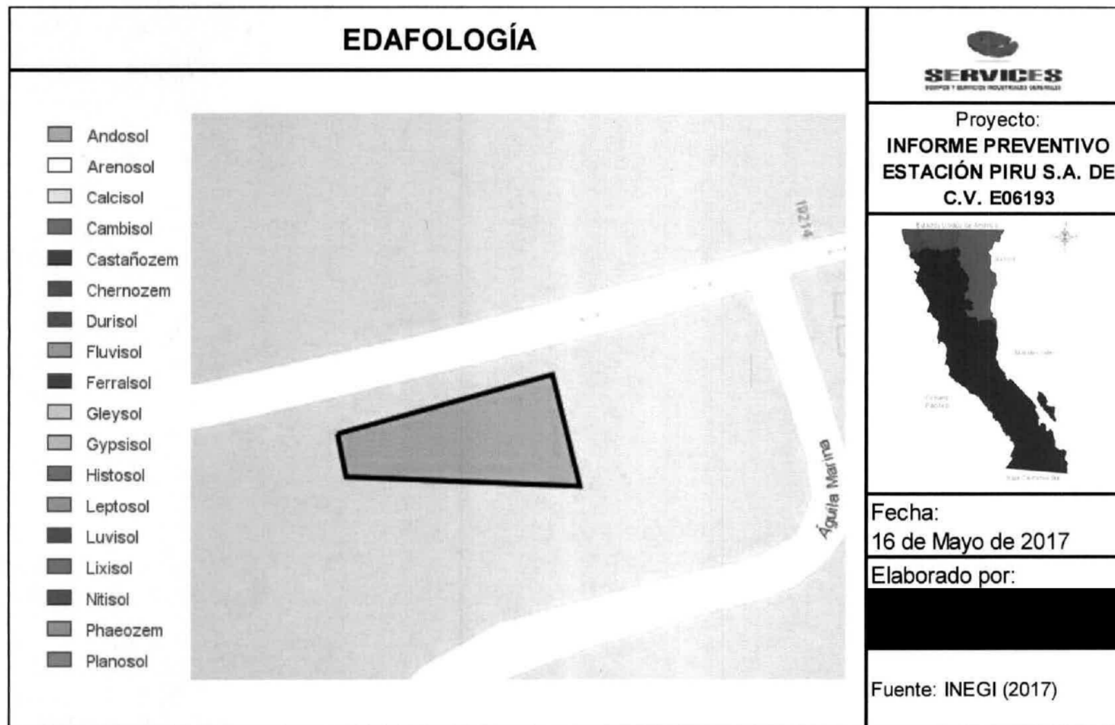
FIGURA 16. EDAFOLOGÍA
