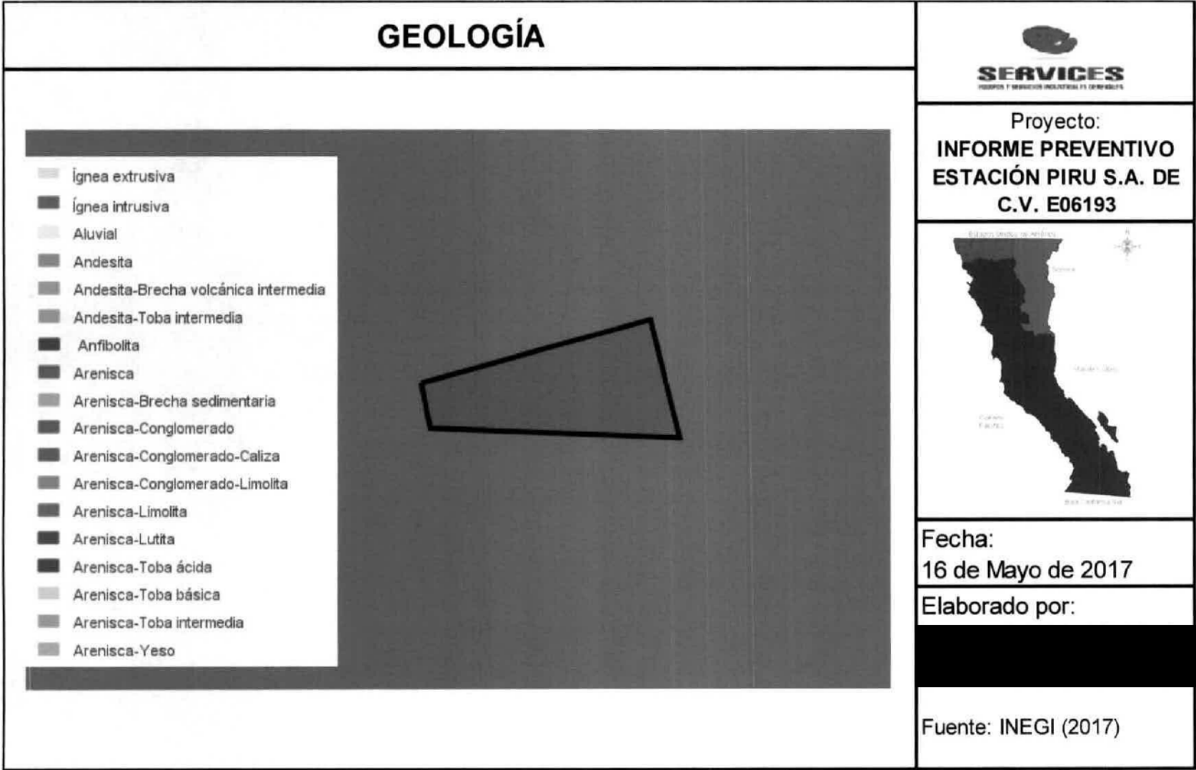
FIGURA 15. GEOLOGÍA
