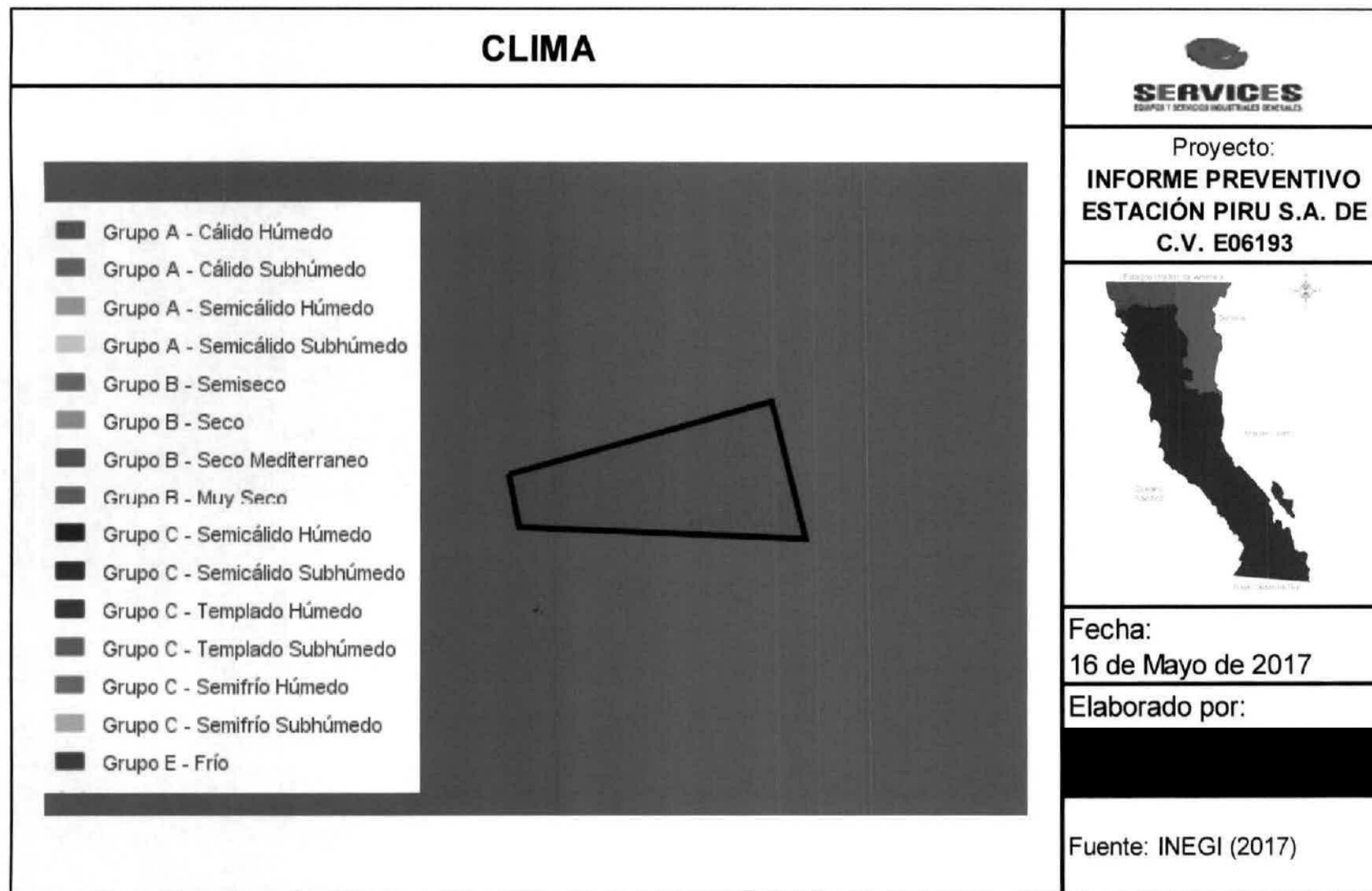
FIGURA 14. CLIMA
