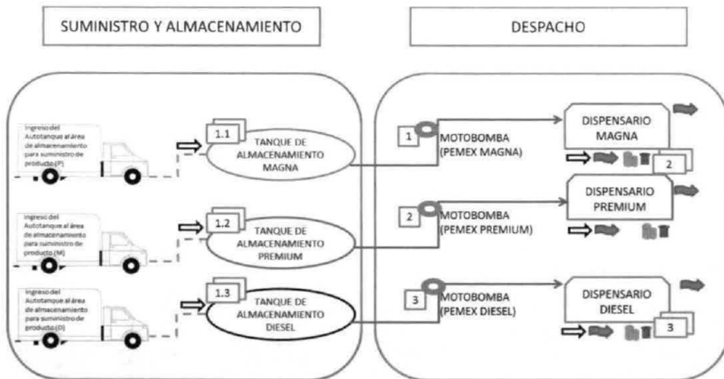
FIGURA 10. DIAGRAMAS TUBOS DE VENDEO
