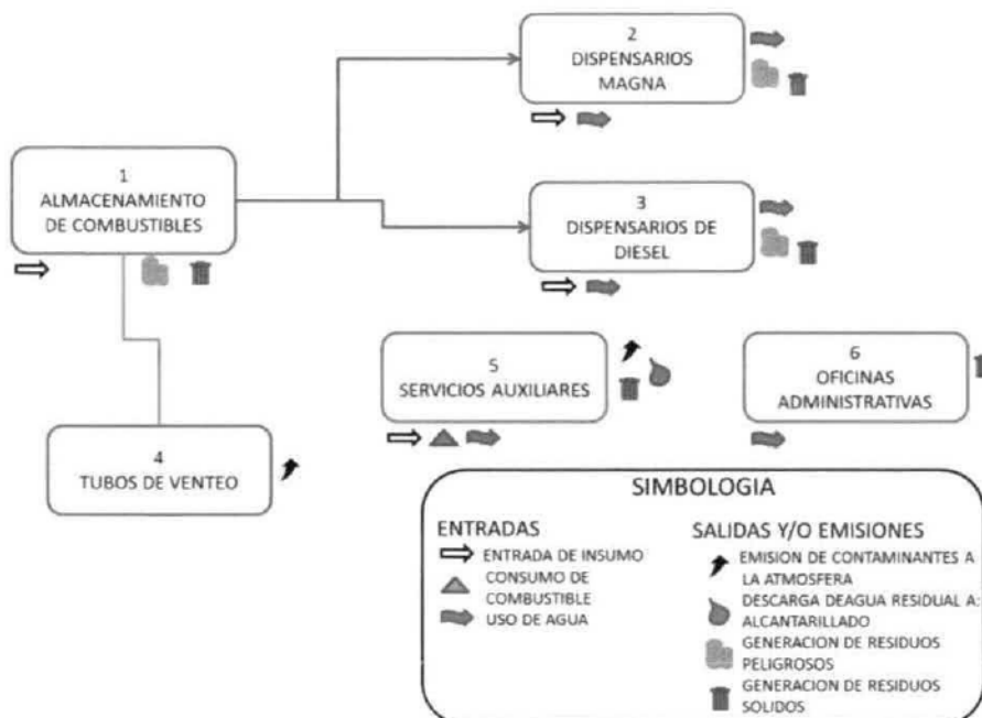
FIGURA 9. DIAGRAMA DE ALMACENAMIENTO
