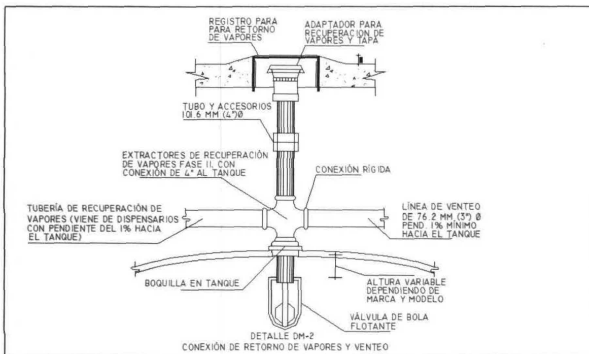
Figura 12. Conexión de retorno de vapores y venteo.
