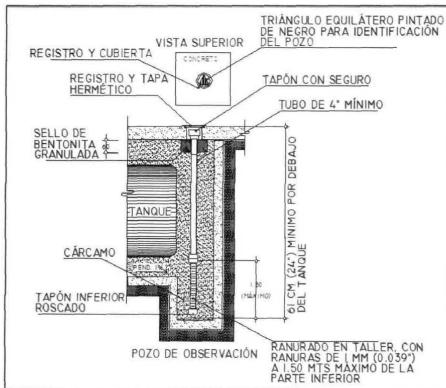
Figura 14. Ejemplo de las características del pozo de observación.
