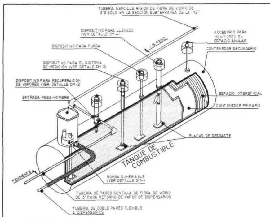
Figura 11. Ubicación de dispositivos en el tanque de almacenamiento.
