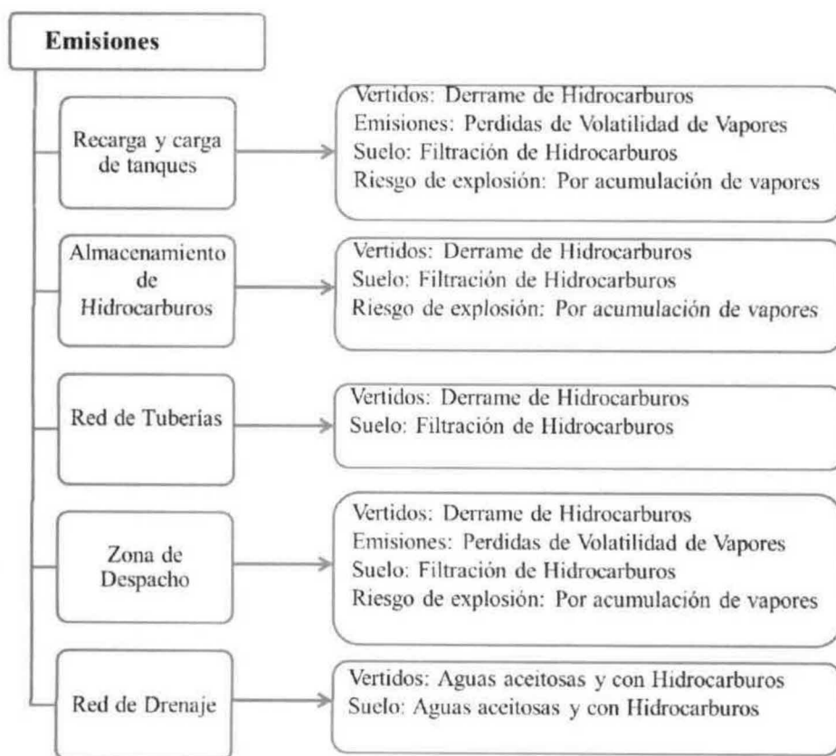
Figura 6. Diagrama de las emisiones en las áreas de las estaciones de servicios.
