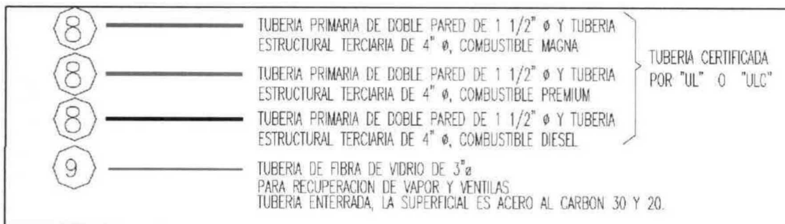
Figura 10. Simbología de líneas de conducción.
