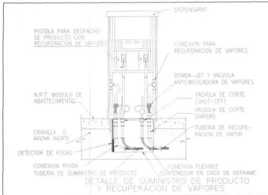
Figura 13. Detalle de suministro de producto y recuperación de vapores.
