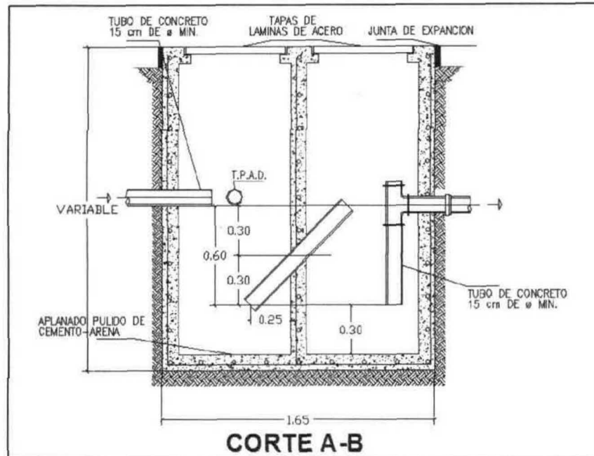
Figura 15. Vistas en planta y en alzado de la Trampa de aceites y combustible.
