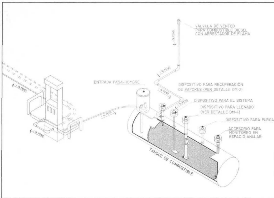
Figura 9. Ejemplo del dispositivo de recuperación de vapores.
