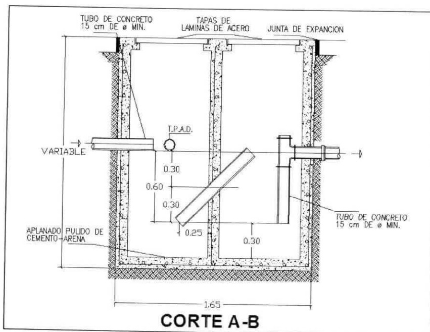
Figura 11. Vistas en planta y en alzado de la Trampa de aceites y combustible.
