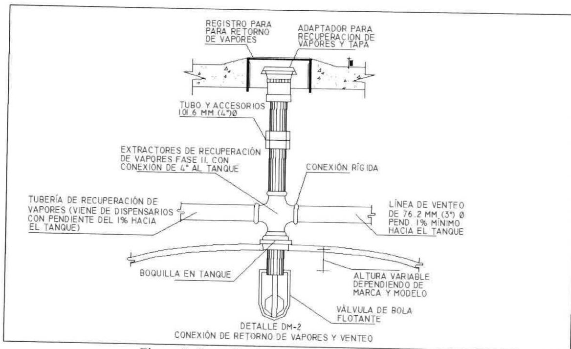
Figura 8. Conexión de retorno de vapores y venteo.
