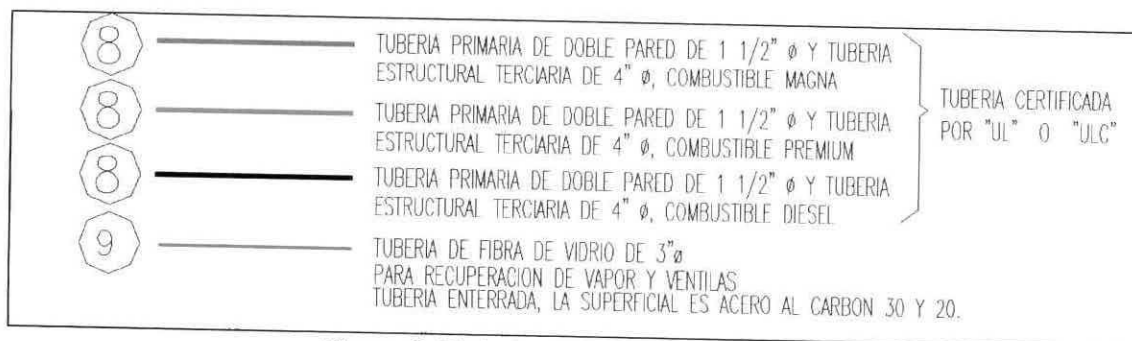
Figura 6. Simbología de líneas de conducción.
