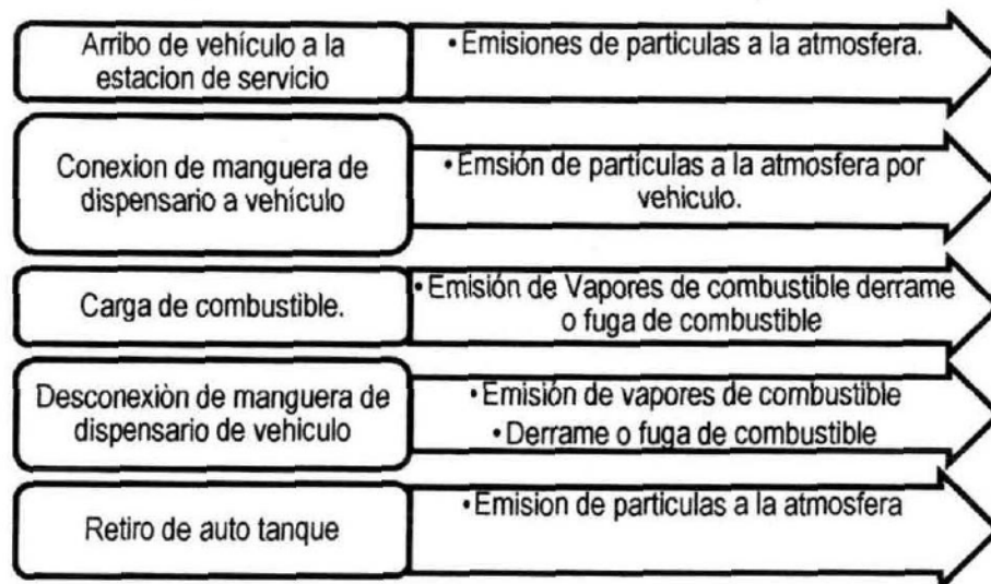
Diagrama 2. Proceso de carga de combustible a vehículos automotores en el área de servicio.
