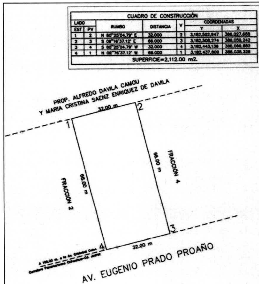
Imagen 7. Dimensiones de la Estación de Servicio ANDOVI.
