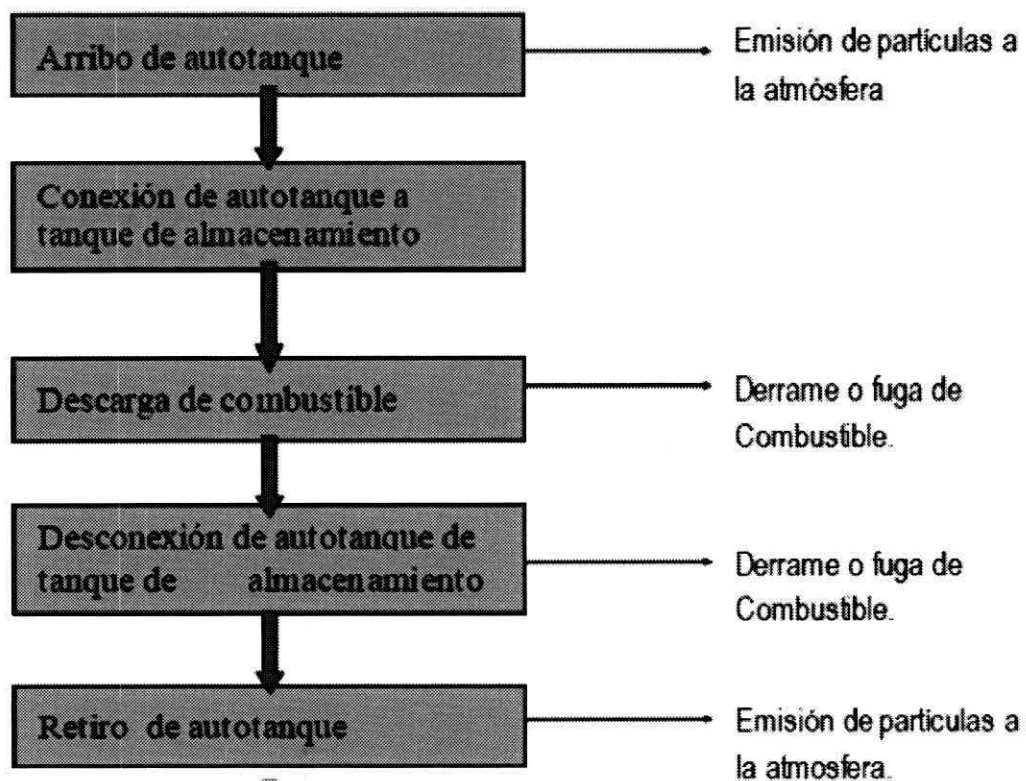
Diagrama 2. Proceso de descarga de combustible del autotank al tanque de almacenamiento
