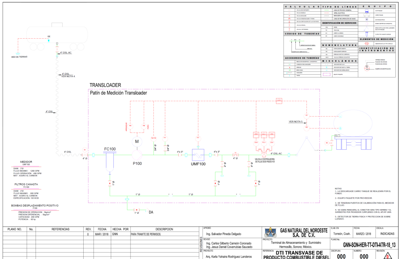
Figura I. 1 DTI de la operación del transloader para descarga de Diesel.
