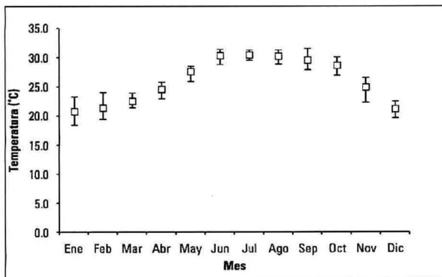
Temperatura promedio mensual (□), con valores mínimos y máximos (-), durante 1995-2010 en Culiacán, Sinaloa. Datos: Estación Meteorológica Escuela de Biología, Universidad Autónoma de Sinaloa.
