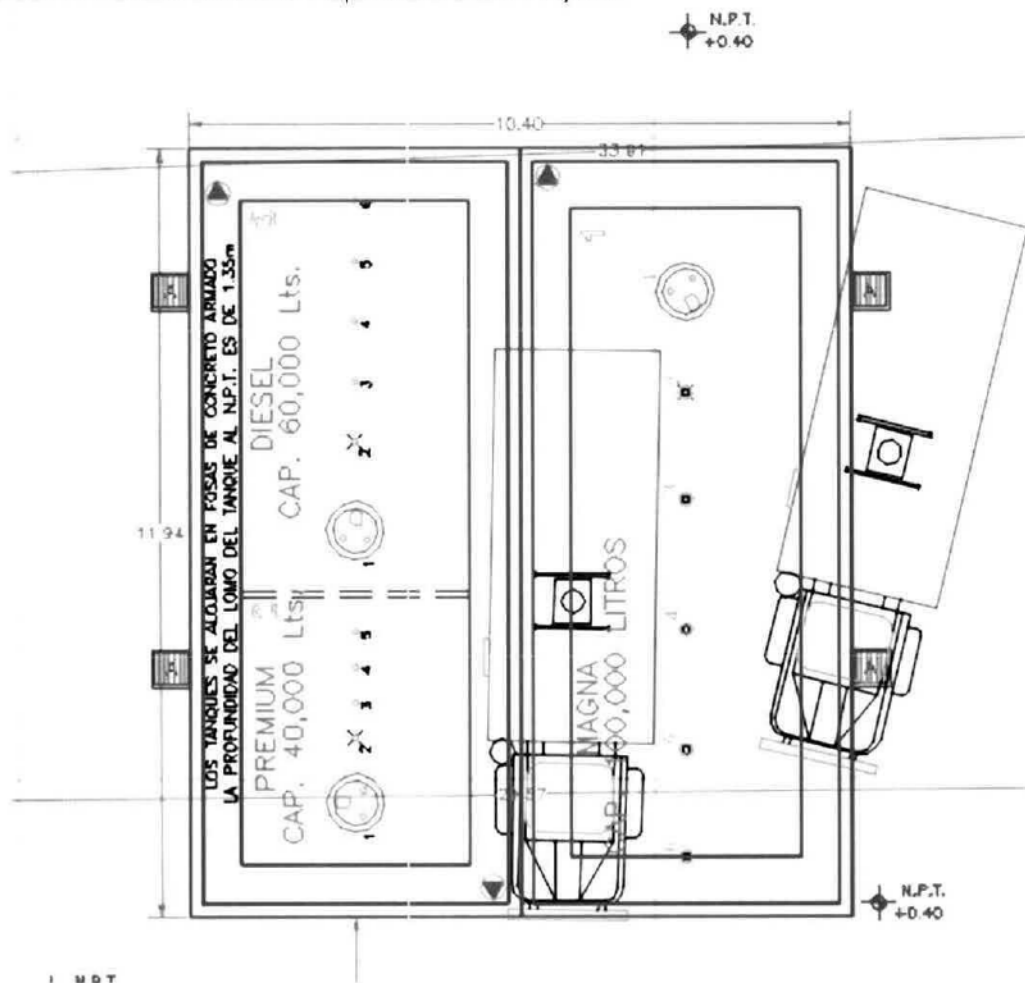
Ilustración 3. Extracto del Plano Arquitectónico del Proyecto
