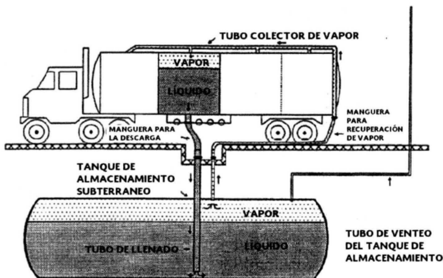
Figura 1. Llenado del almacén subterráneo.
