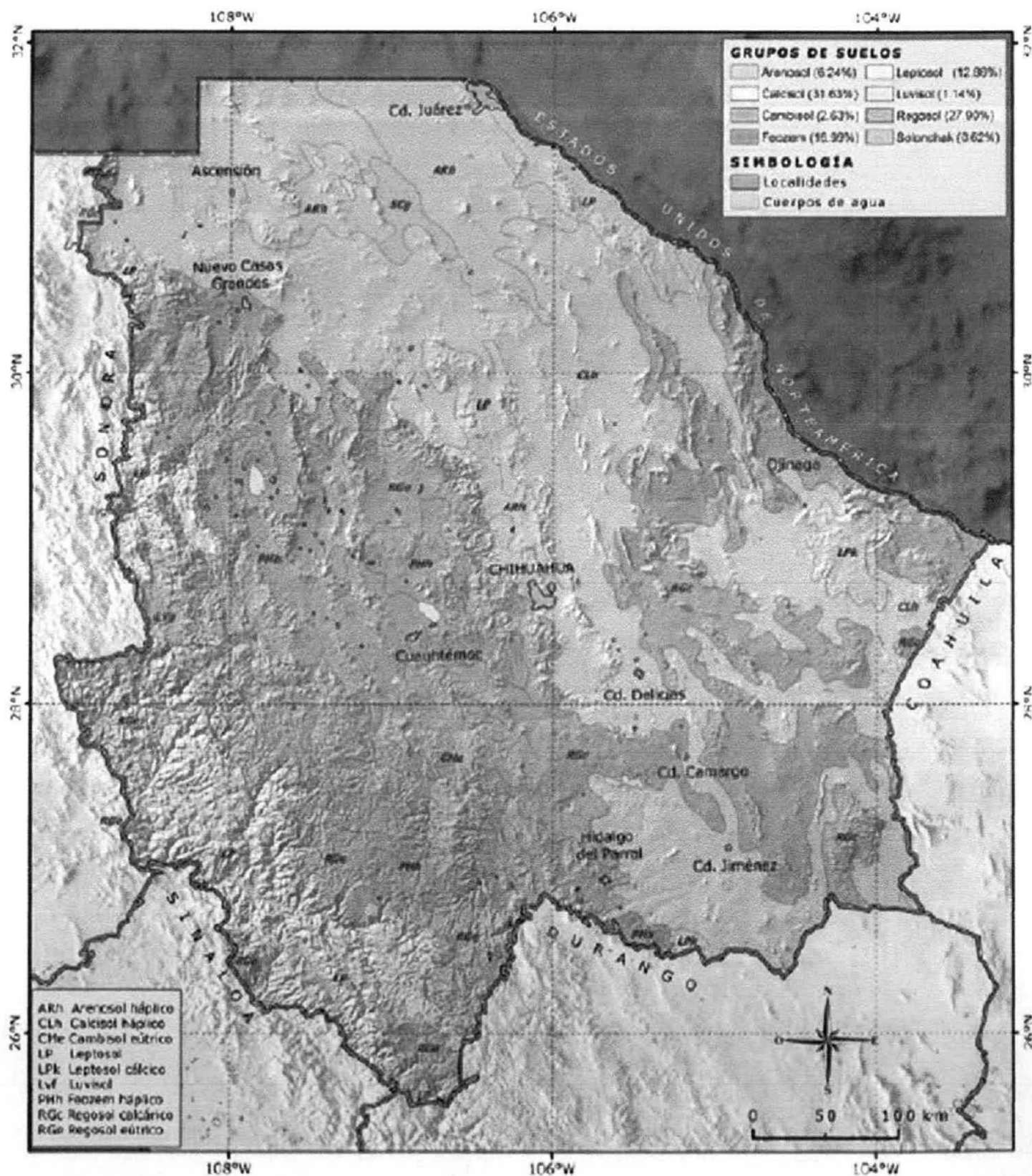
Figura 21. Edafología.
