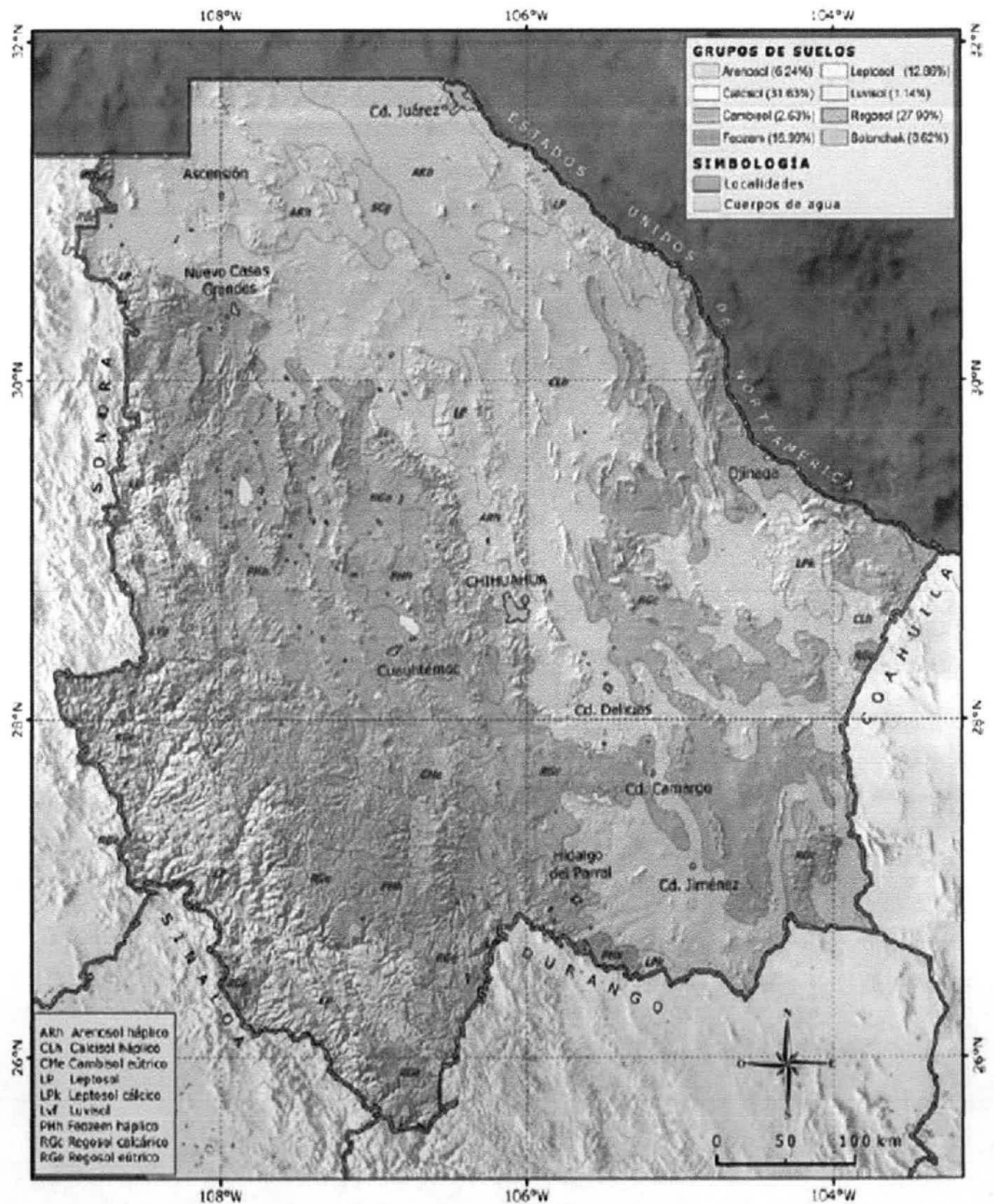
Figura 21. Edafología.
