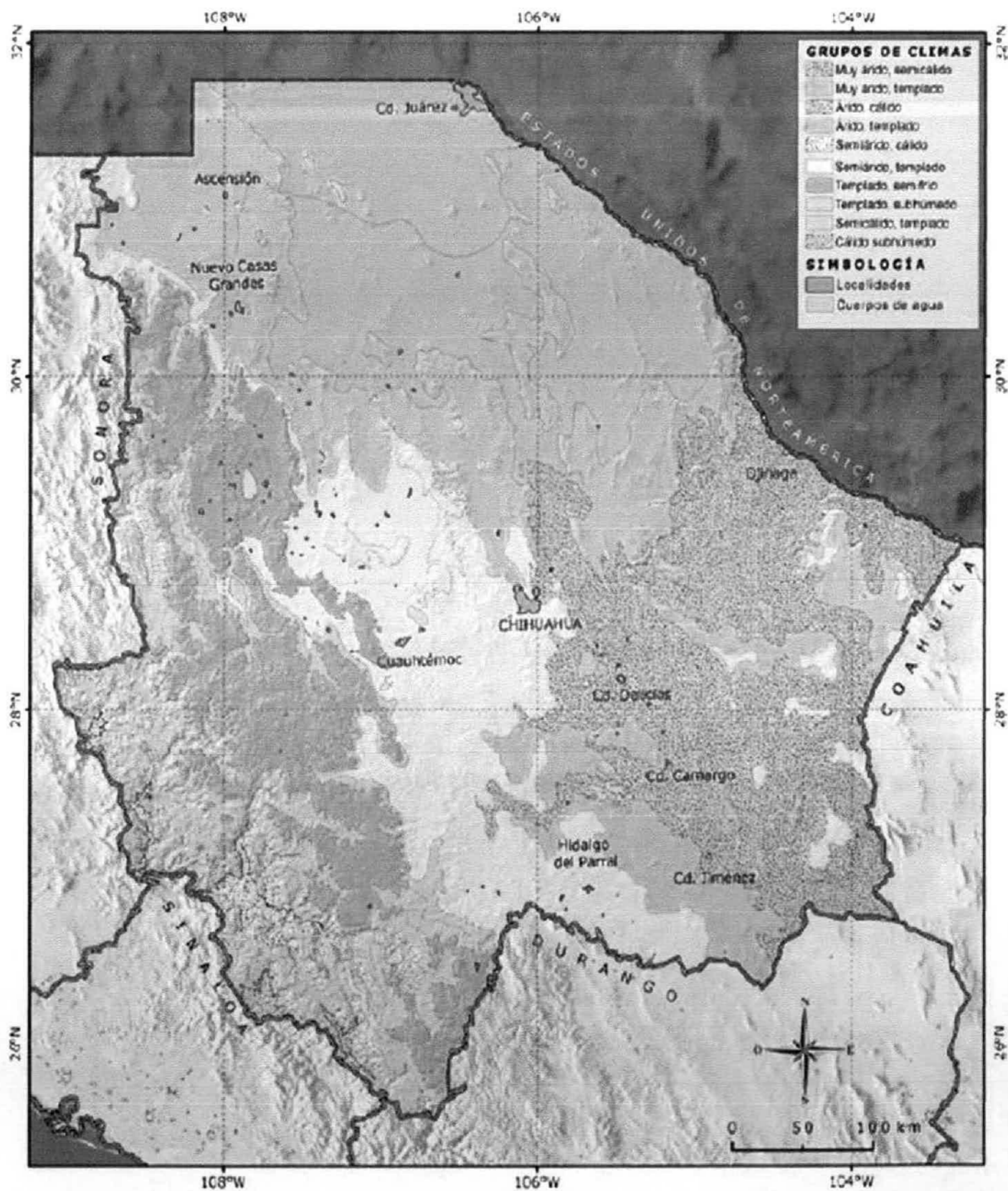
Figura 20. Clasificación climática.
