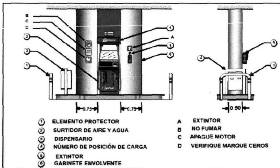
Imagen 7. Muestra de los distintos componentes de que consta cada una de las islas para el despacho de combustibles en la estación de servicio. Todo este equipamiento está adecuado a las especificaciones exigidas por PEMEX.
