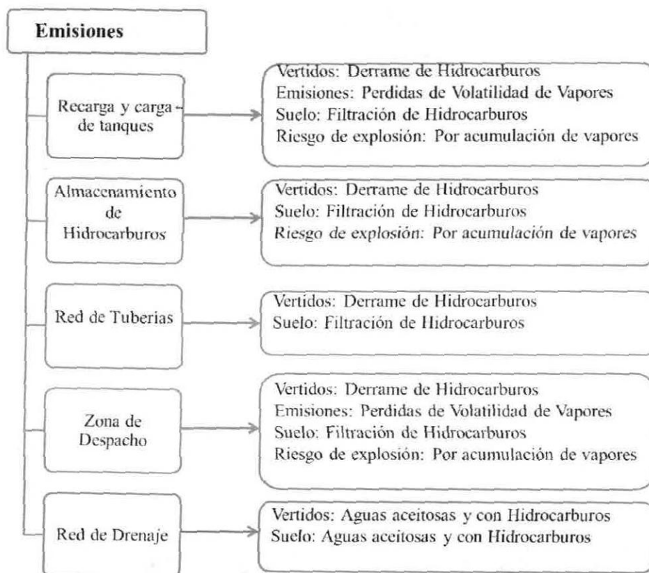
Figura 3. Diagrama de las emisiones en las áreas de las estaciones de servicio.
