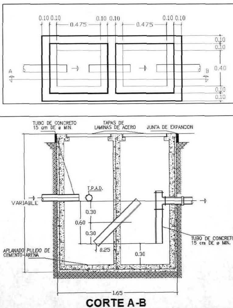
Figura 11. Vistas en planta y en alzado de la Trampa de aceites y combustible.
