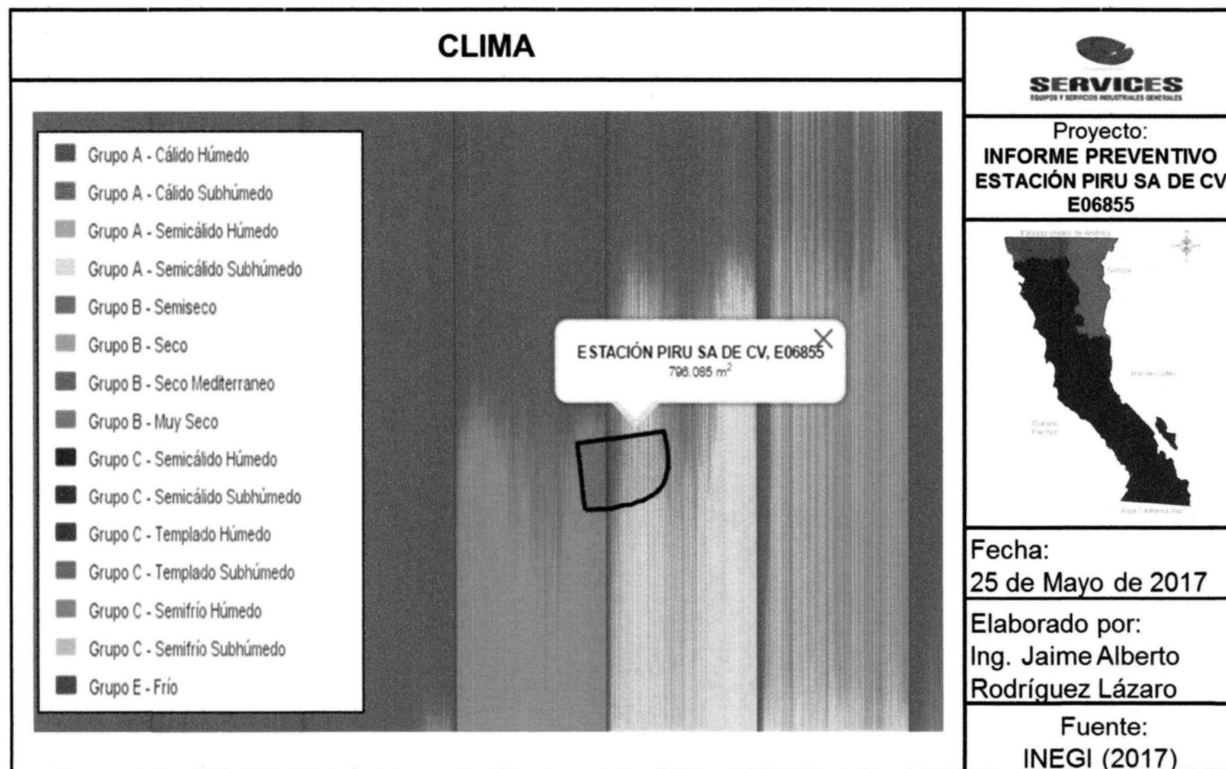
FIGURA 14. CLIMA
