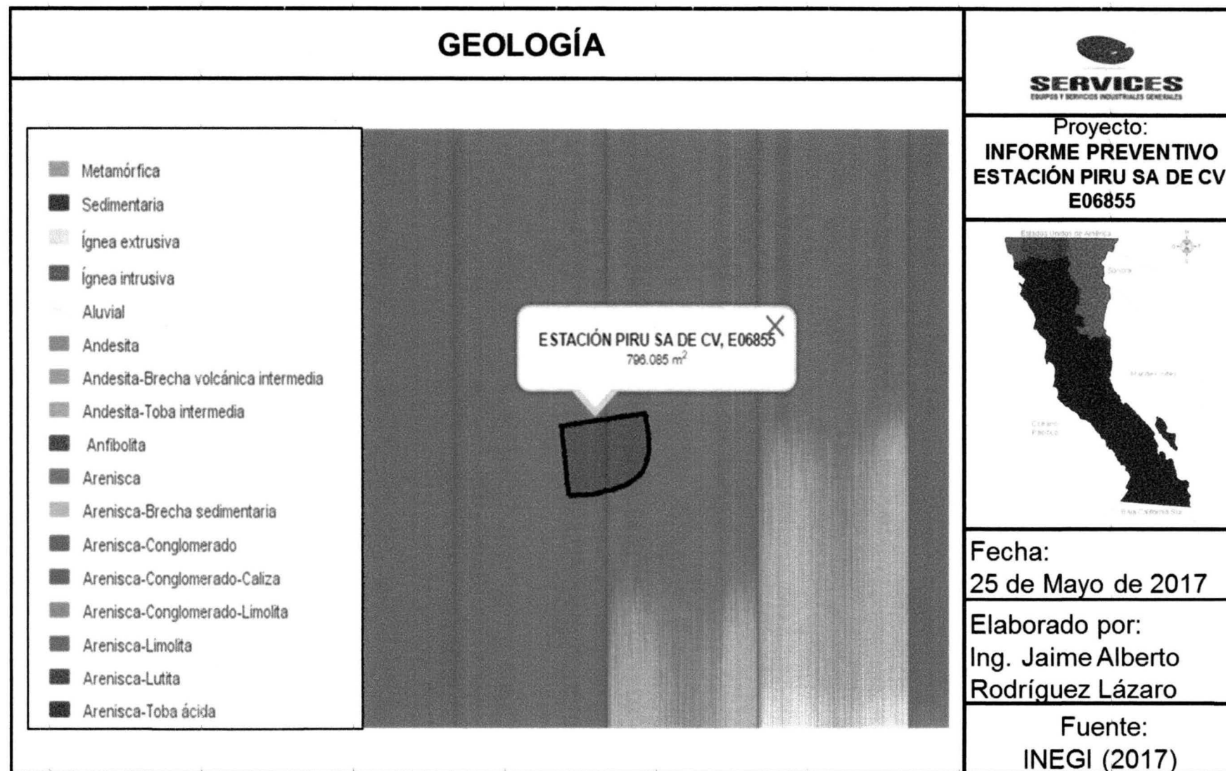
FIGURA 15. GEOLOGÍA
