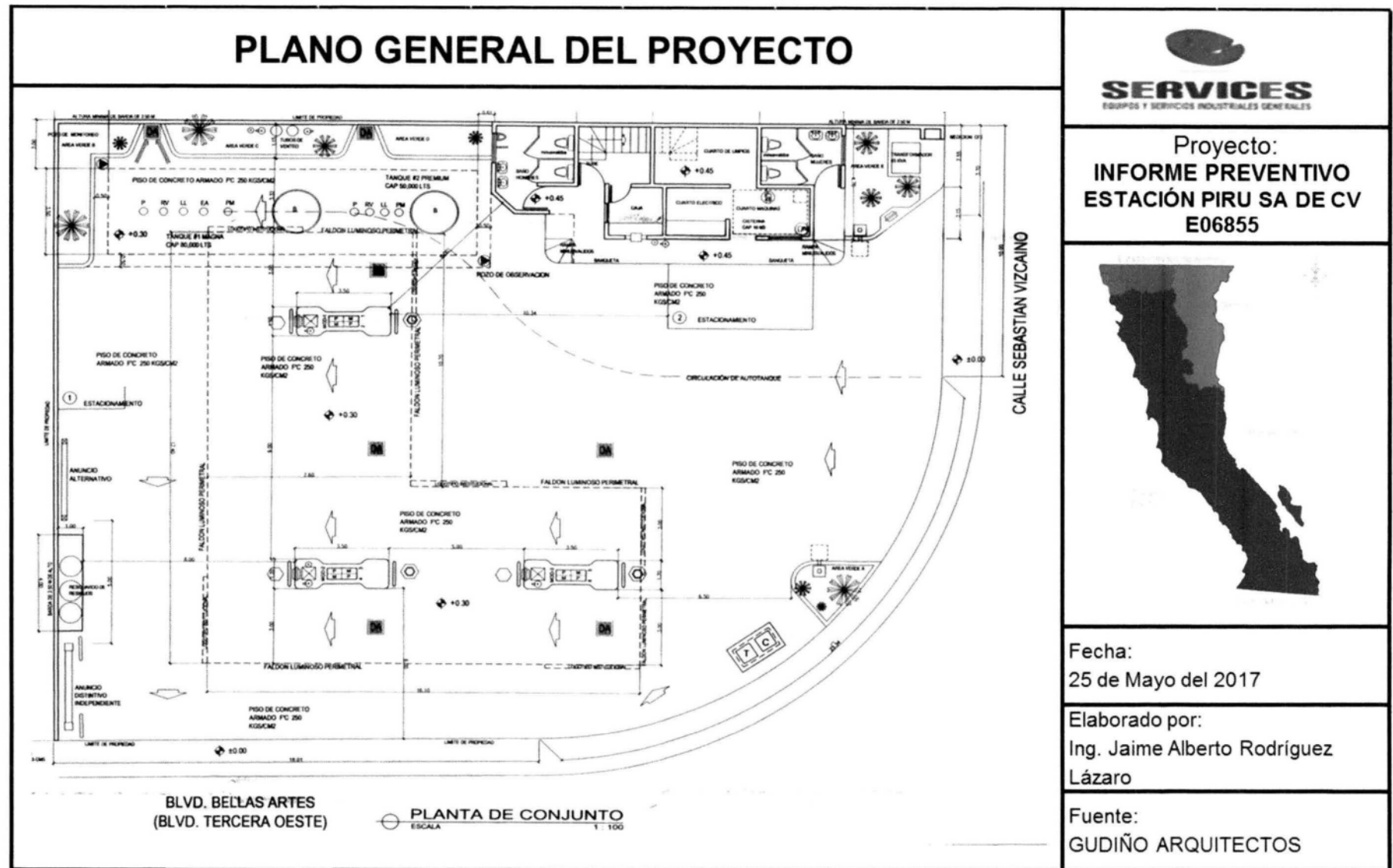
FIGURA 7. PLANO GENERAL DEL PROYECTO.
