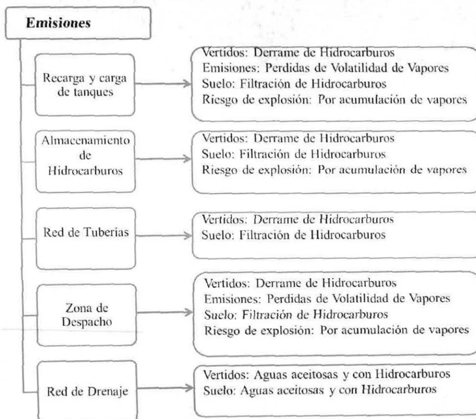
Figura 7. Diagrama de las emisiones en las áreas de la estación de servicios.
