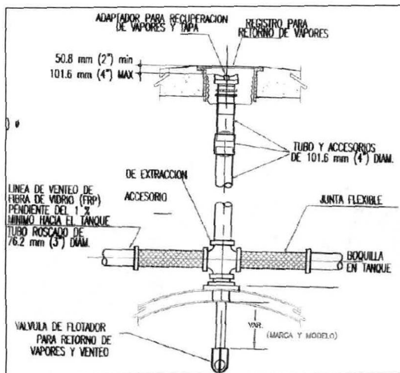
Figura 12. Detalles del sistema de recuperación de vapores.
