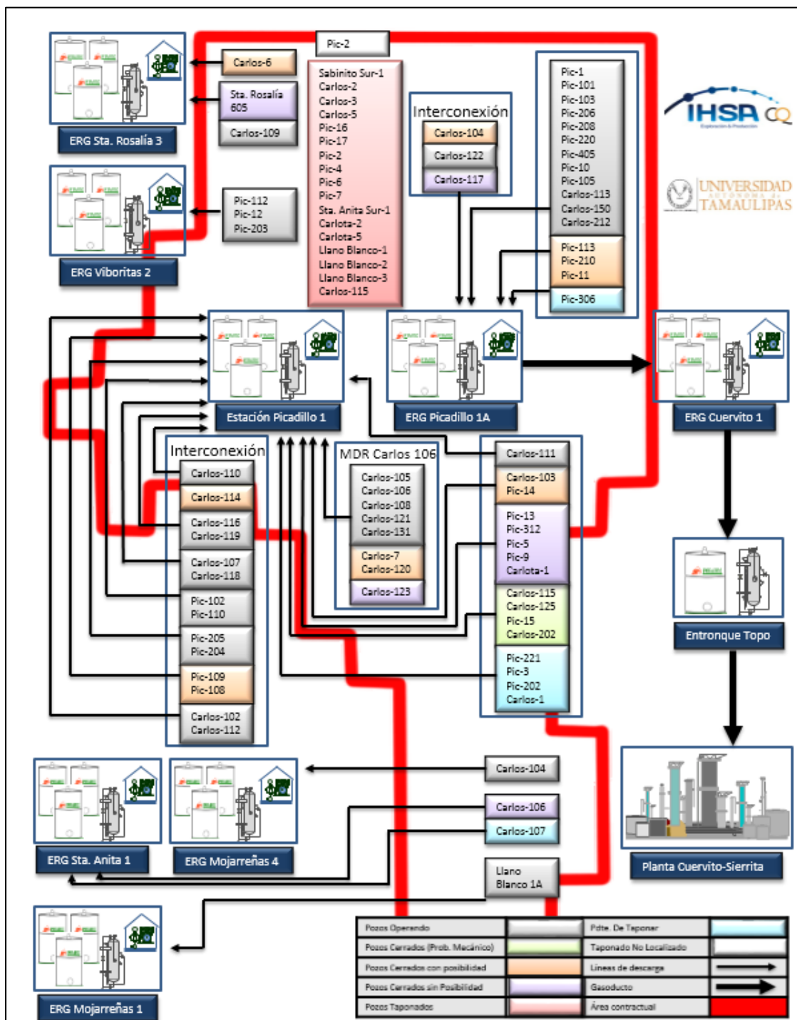
Figura III-4.- Diagrama de flujo de proceso del Área Contractual BG-01.
