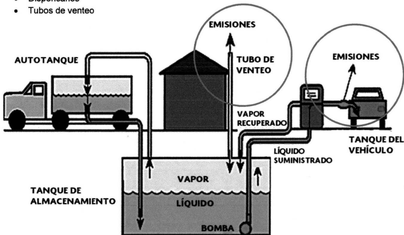
Figura 1. Lugares de emisiones de contaminantes a la atmosfera en una estación de servicio
