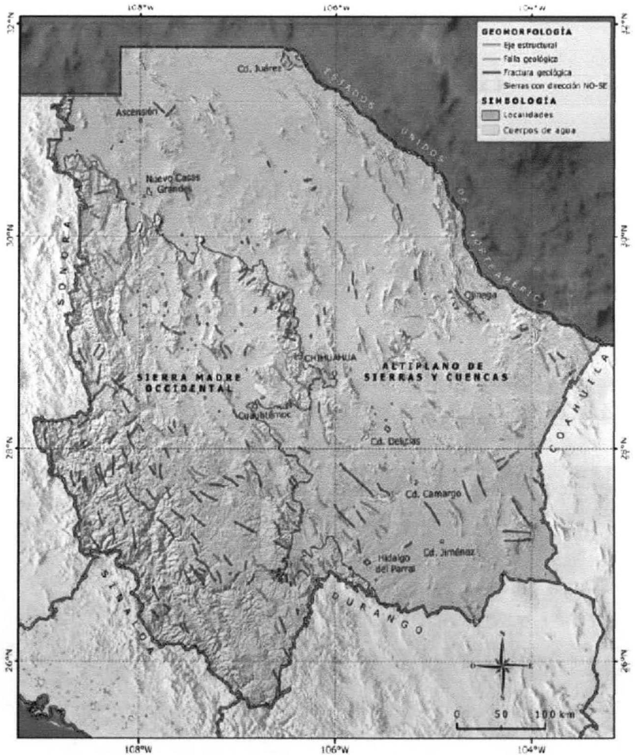
Figura 5. Regiones geomorfológicas.
