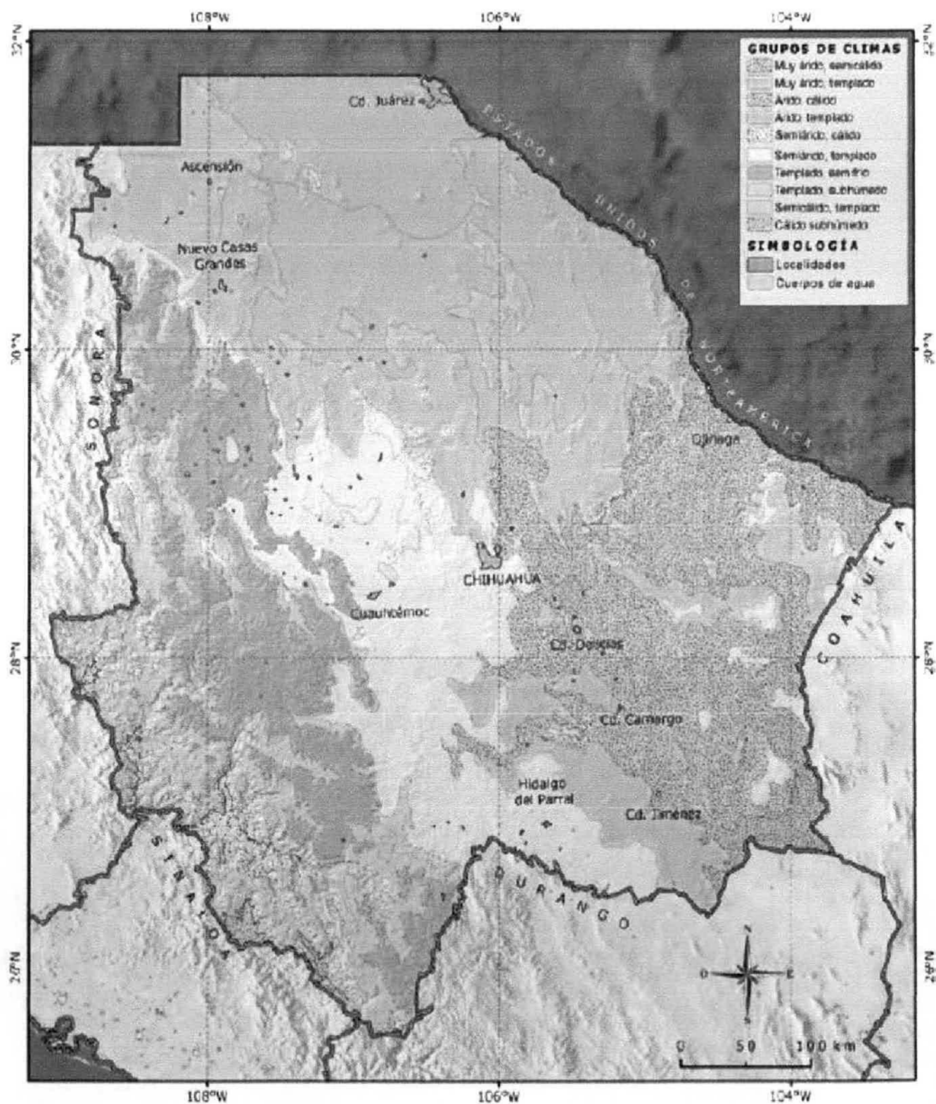
Figura 20. Clasificación climática.
