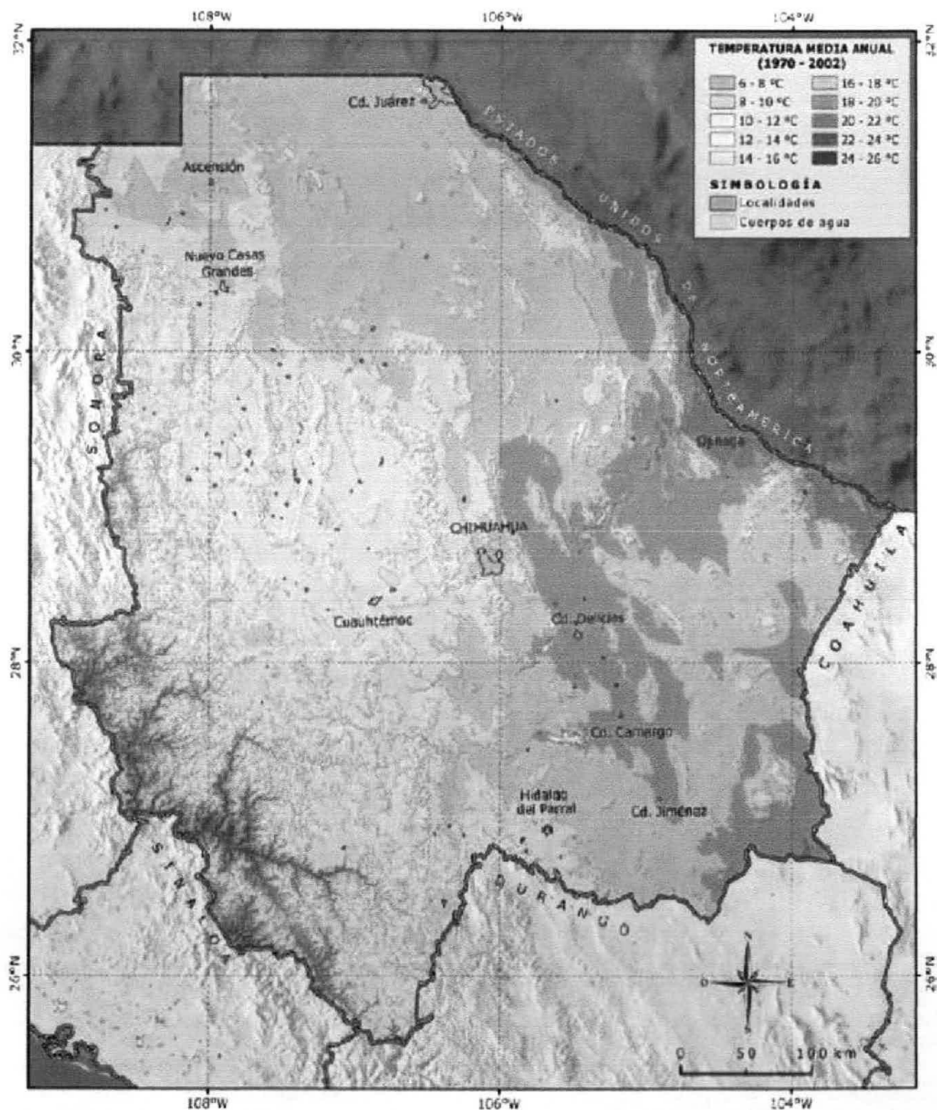
Figura 19. Distribución espacial de la temperatura promedio anual histórica. Periodo analizado 1970-2001.
