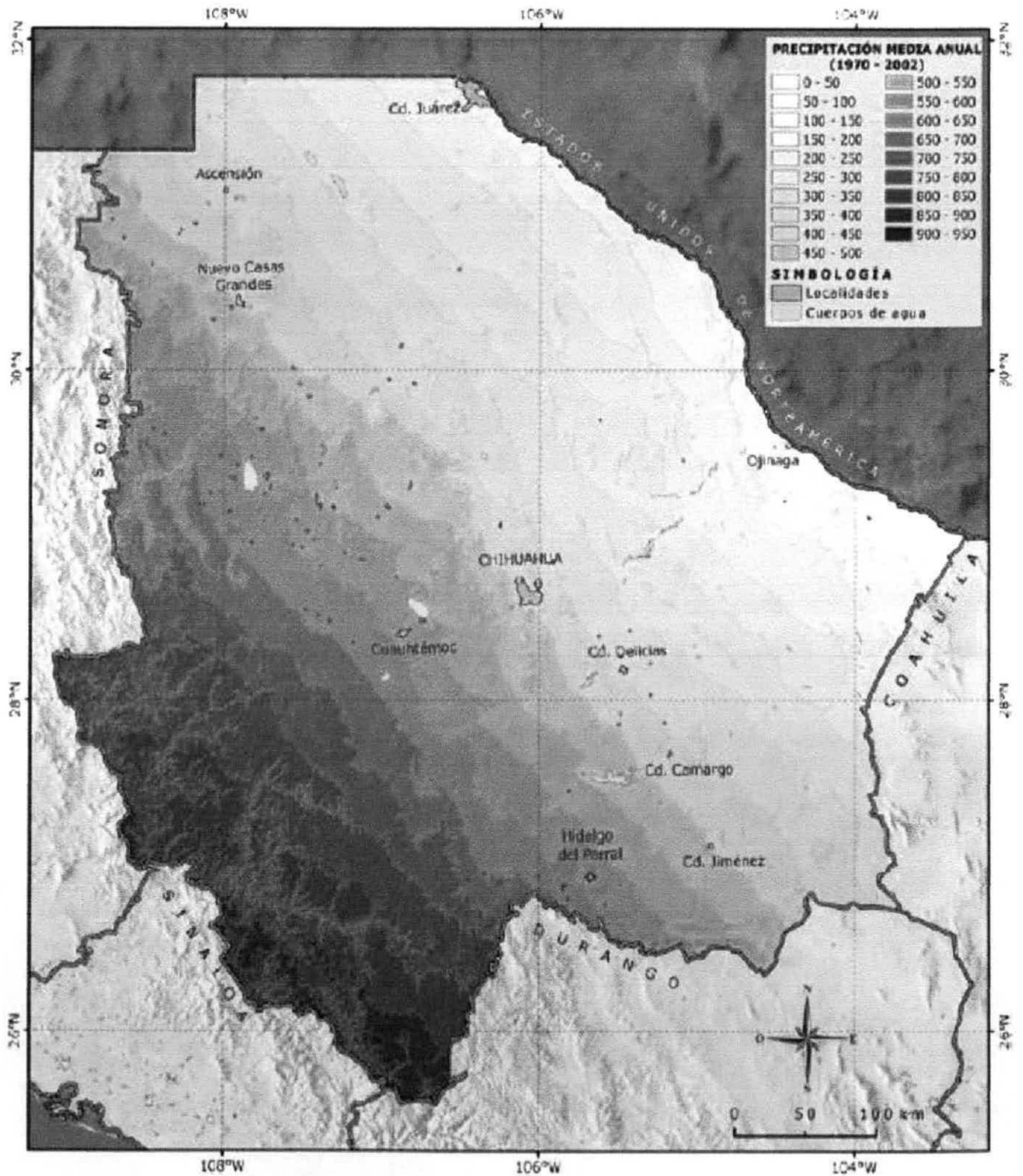
Figura 17. Distribución espacial de la precipitación media anual histórica. Periodo analizado 1970-2001.
