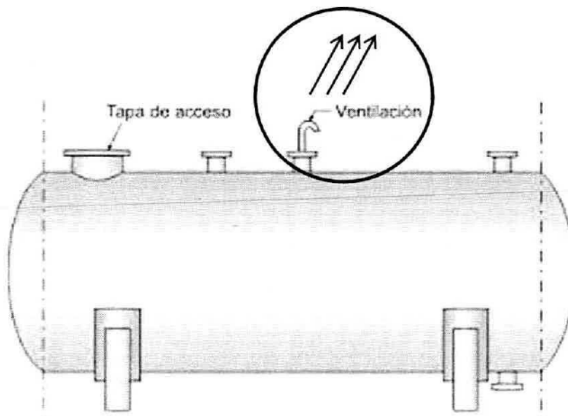
Figura 1. Lugar de emisión de contaminantes a la atmosfera en un tanque estacionario
