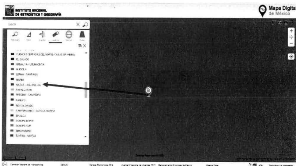
Figura 14. Cuencas y Subcuencas Hidrológicas
