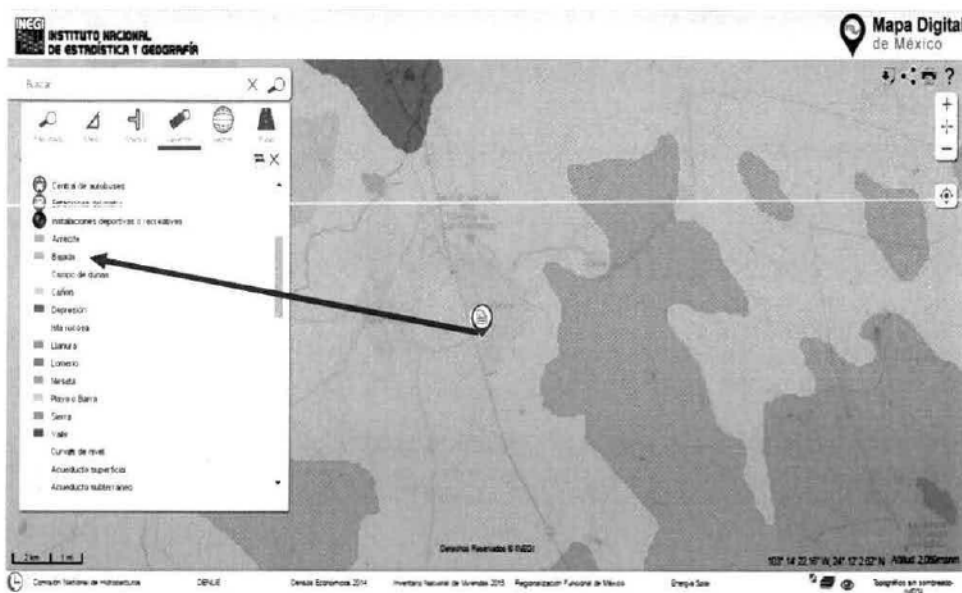
Figura 12. Imagen de la Geomorfología del Mpio.
