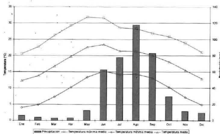
Figura 39. Distribución de la precipitación y temperatura de la estación Juan Aldama, Juan Aldama.
