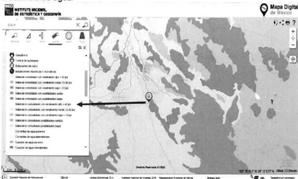
Figura 13. Imagen Hidrología del Municipio
