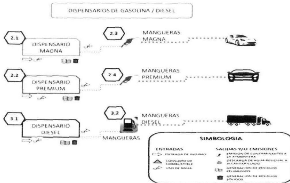
2 Y 3) DIAGRAMA DISPENSARIOS DE GASOLINA / DIESEL
